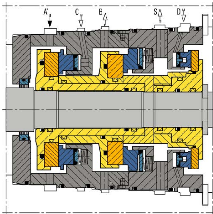
CobaDGS tandem arrangement.
